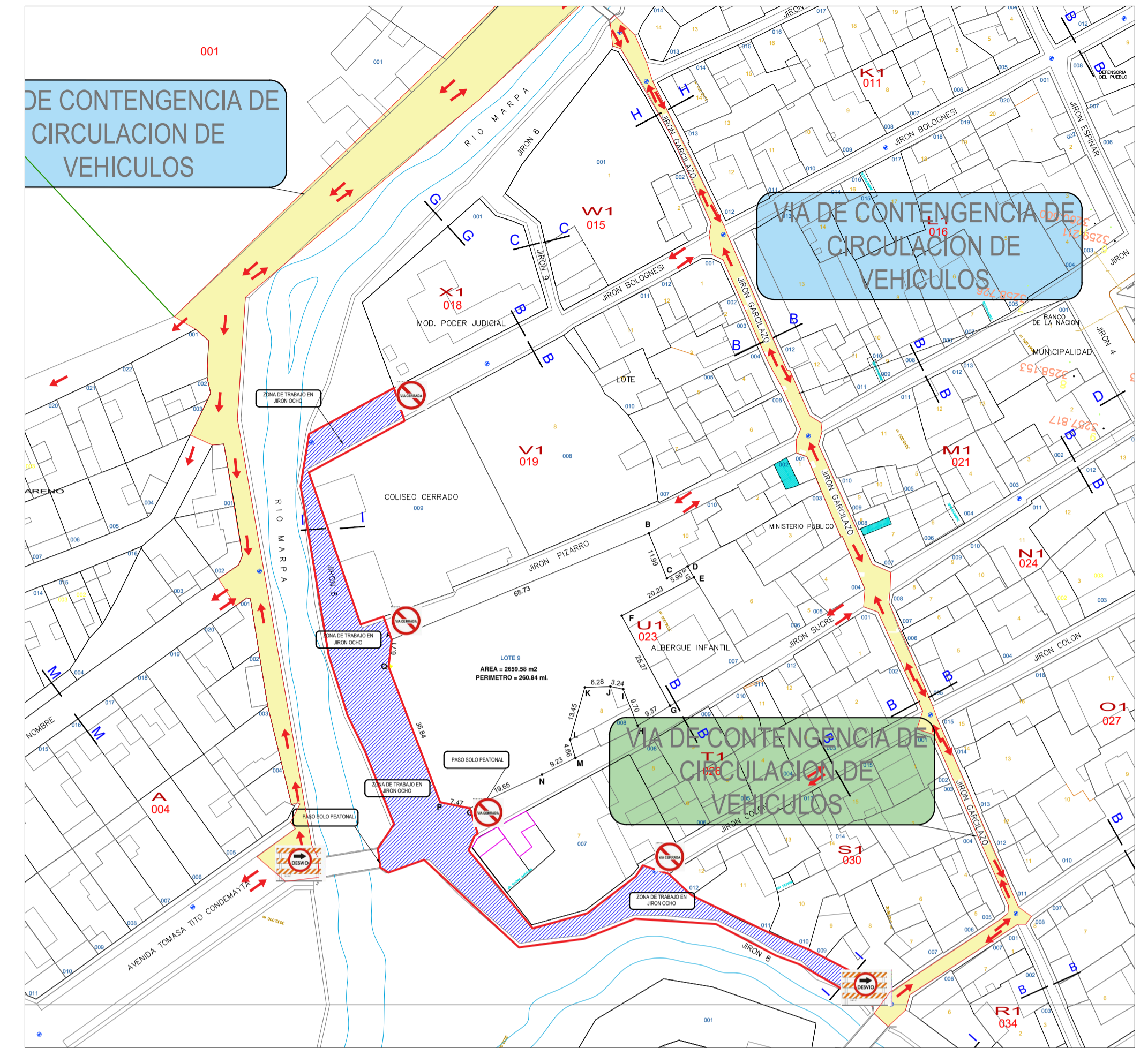
PLANO DE UBICACION DE DESVIO DE VIAS ESCALA 1:1000
